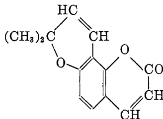
Seselin
