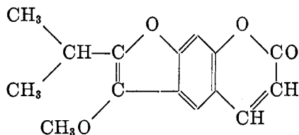
Peucedanin
