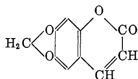
Ayapin
