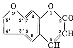
I Psoralene
