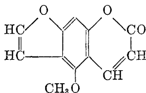
Bergaptene
