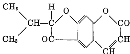
Oreoselone
