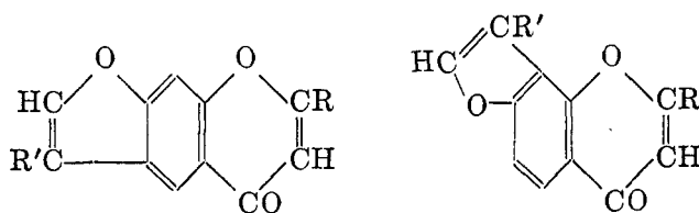
Furanochromones
